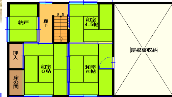
【2階間取図】
